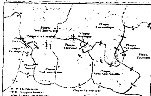
fig.D : mouvements des plaques tectoniques
