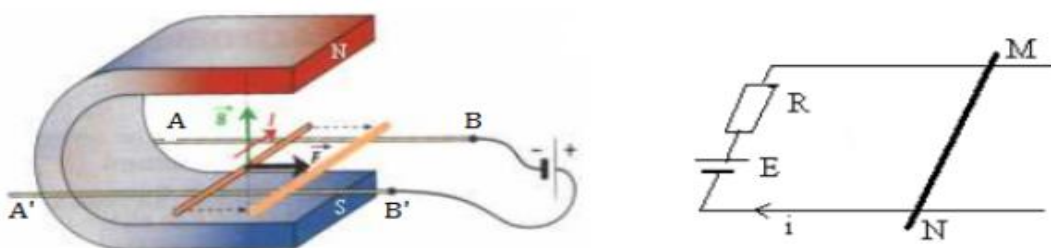
Figure 3.5 : Dispositif expérimental
