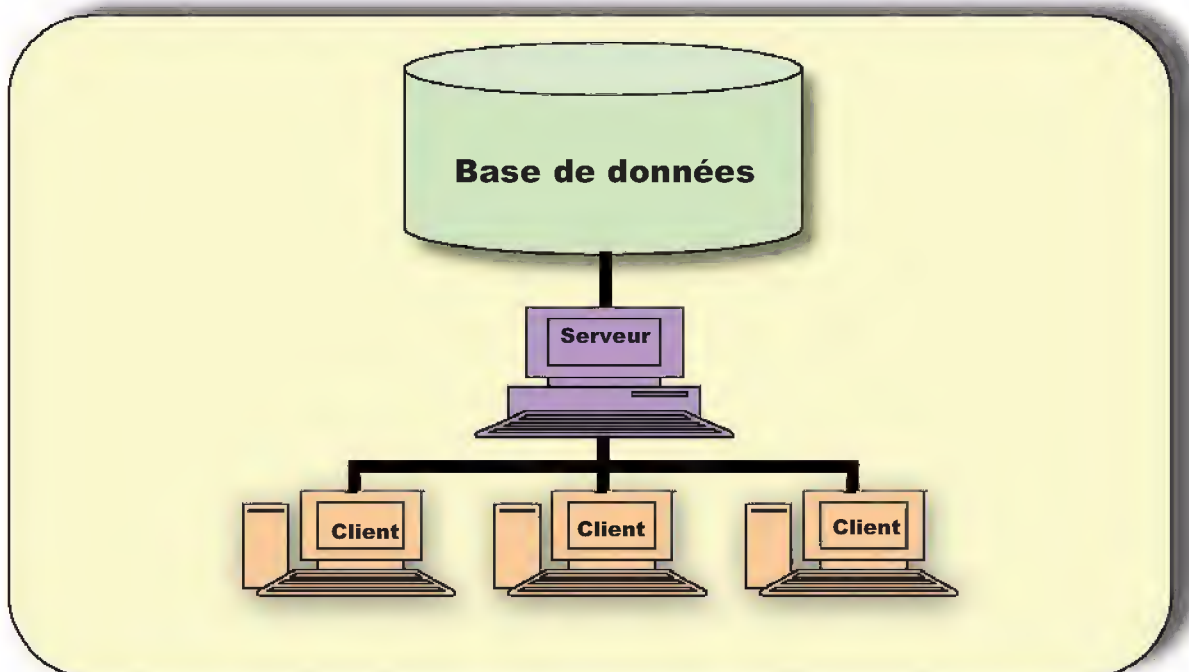
Figure 1.1 : Une base de données dans une architecture client/serveur.
