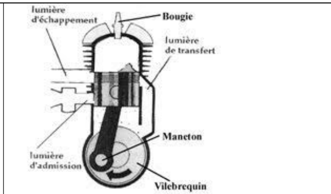
Figure b) moteur à deux temps
